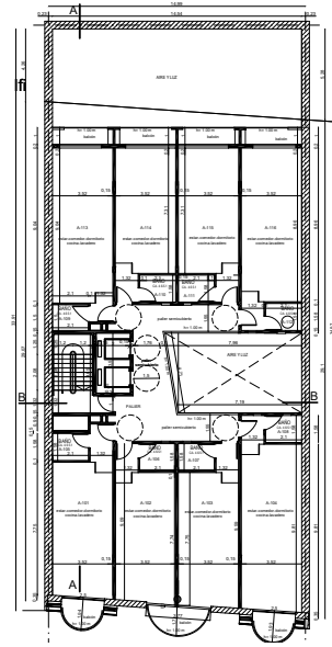
Planta 1er piso
