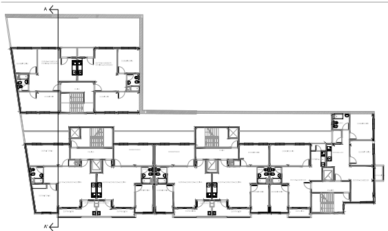
Planta 1er.PISO
