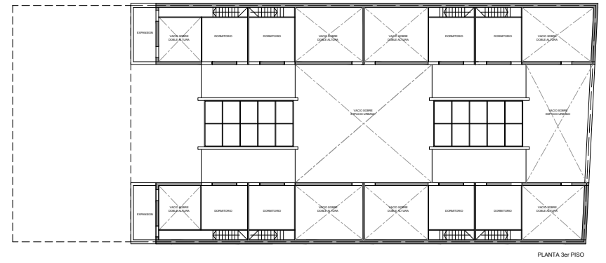
Planta 3er piso
