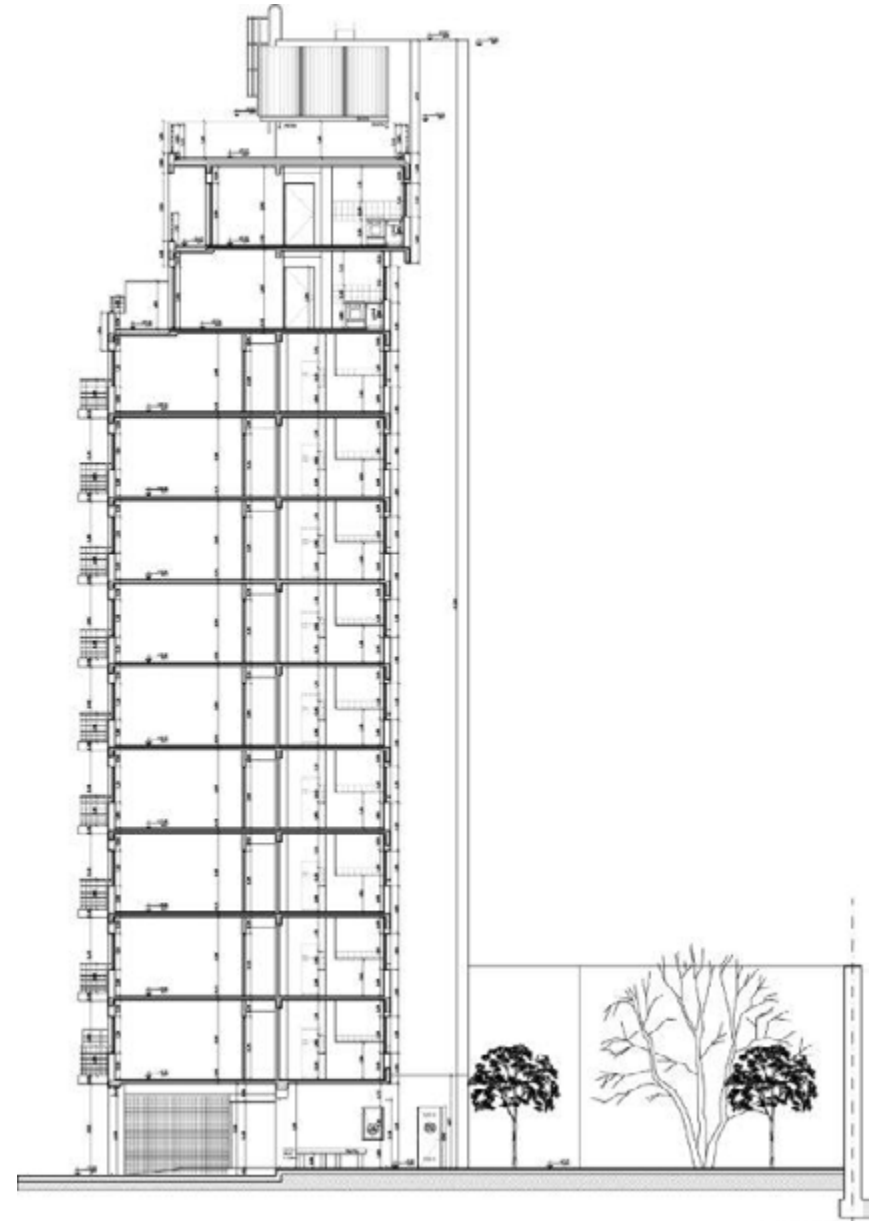
Corte
