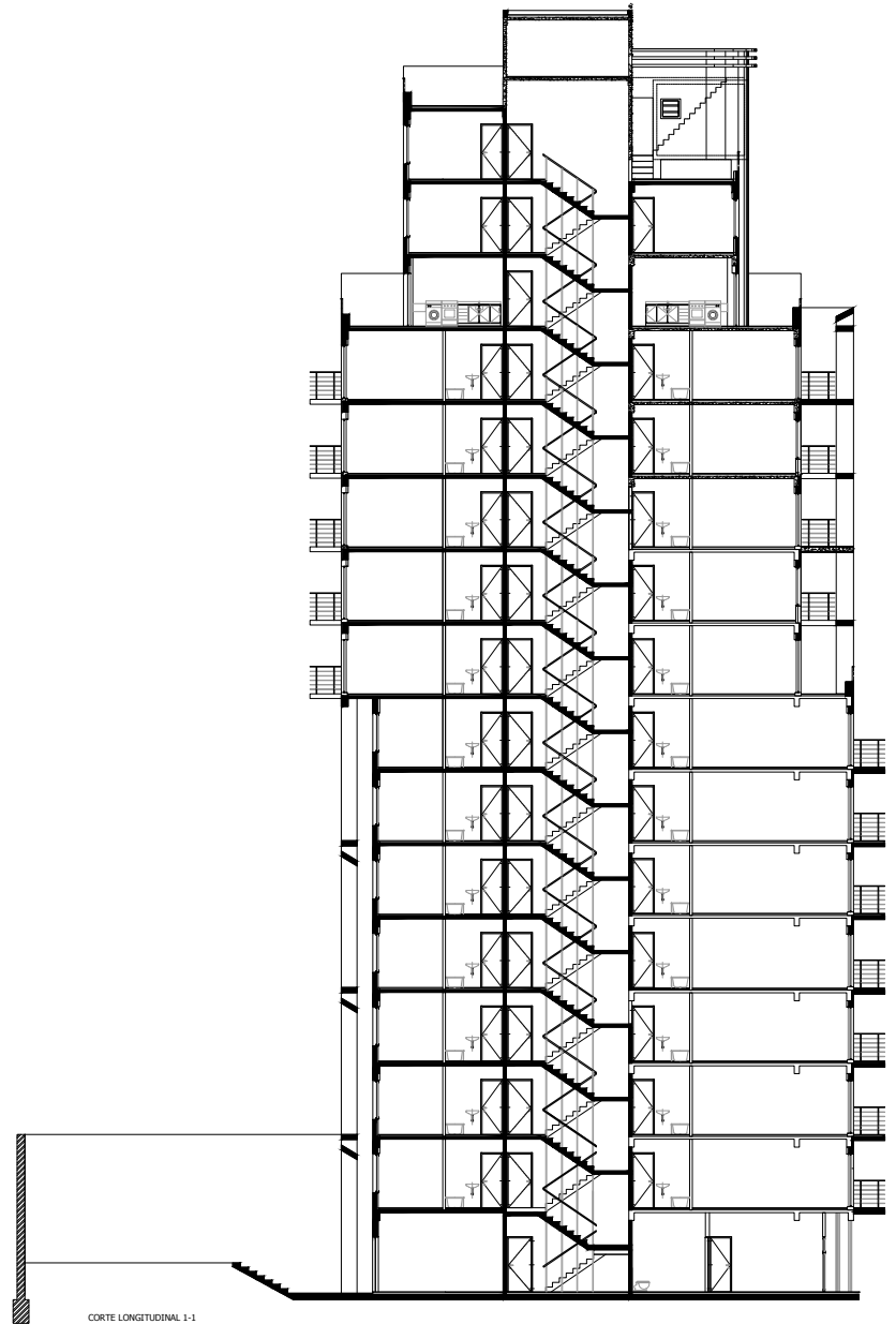
CORTE LONGITUDINAL 1-1
