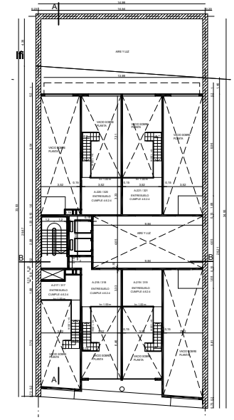
Planta entrespiso 2do y 3er piso
