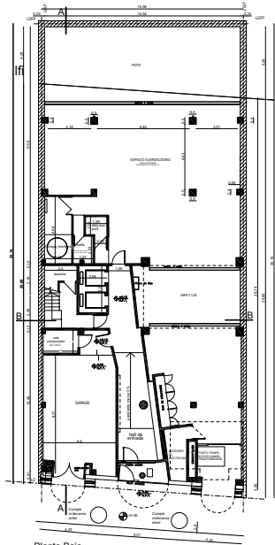
Planta baja
