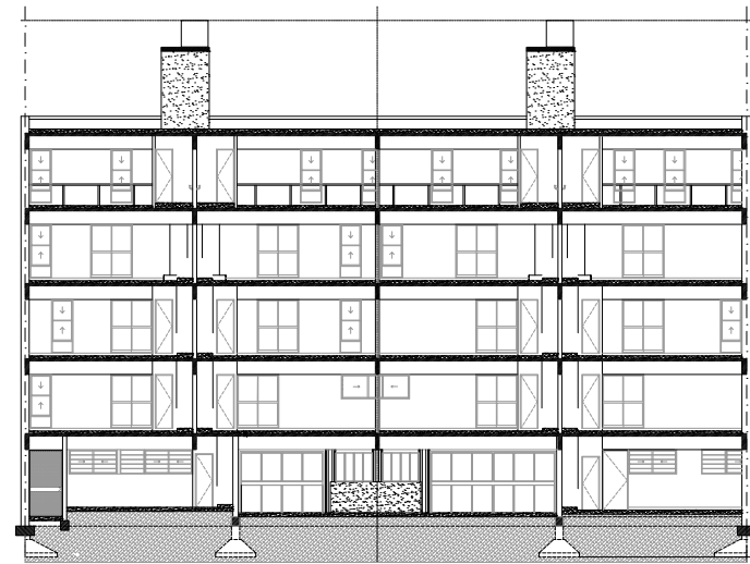
Corte longitudinal C-C
