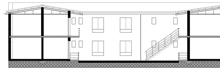
CORTE A-A
