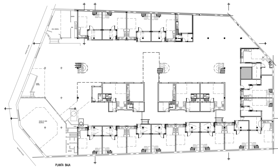
Planta baja
