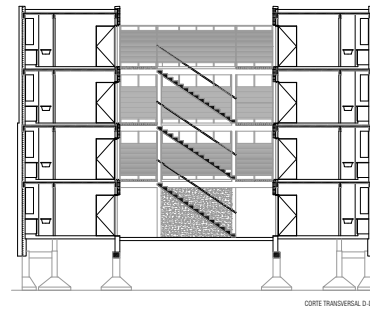
Corte Transversal D-D
