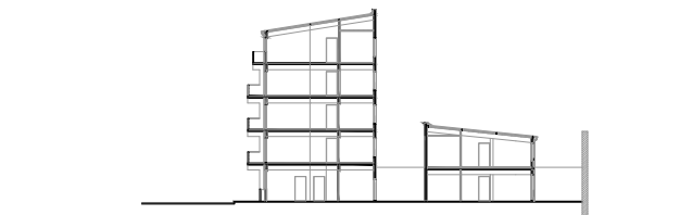
Corte A-A
