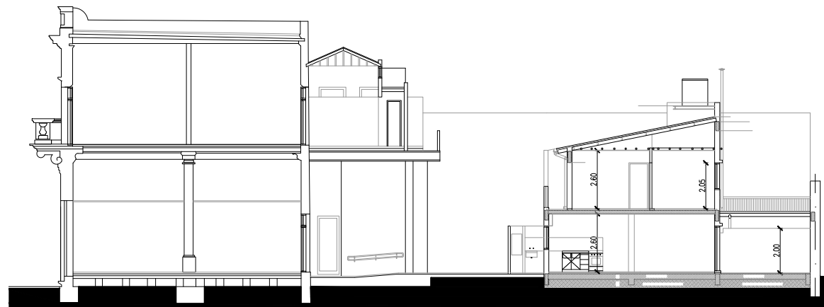
Cortes
