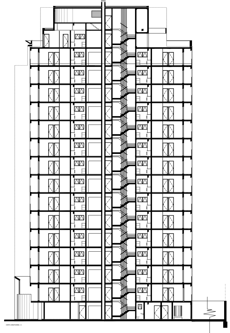
Corte longitudinal
