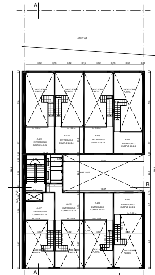
Planta entrespiso 4to piso
