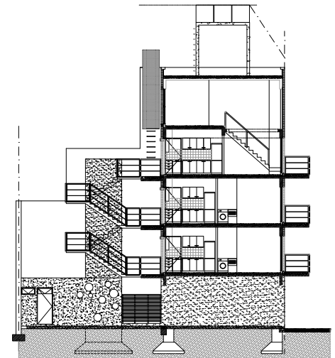
Corte longitudinal B-B
