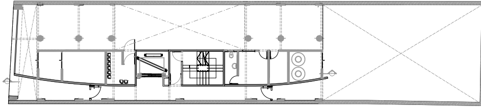
Planta baja
