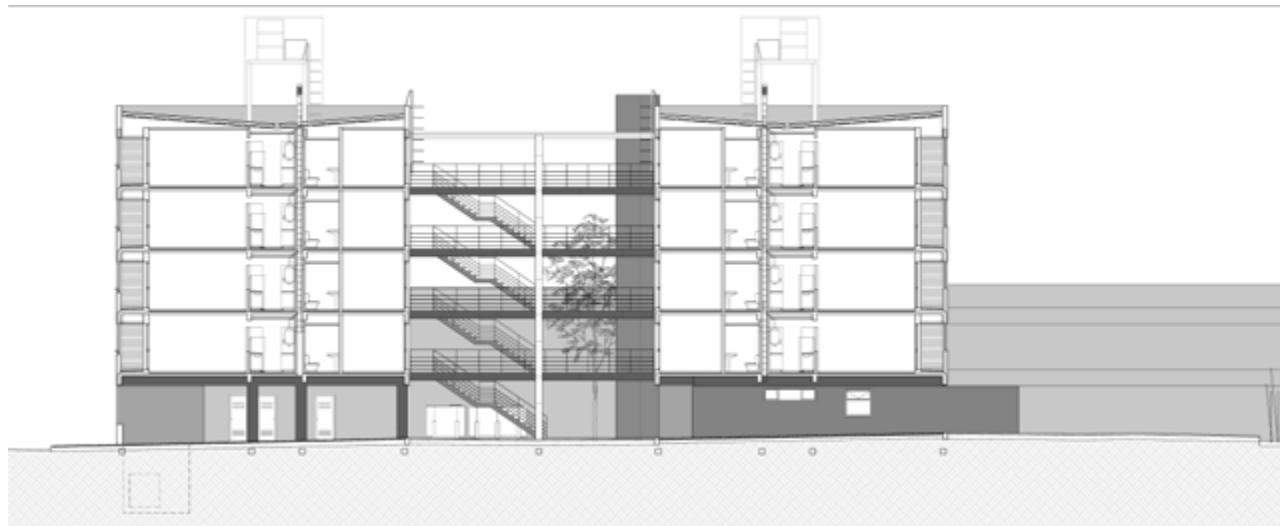
Corte
