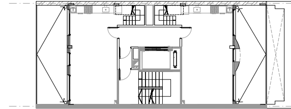
Planta 13er piso
